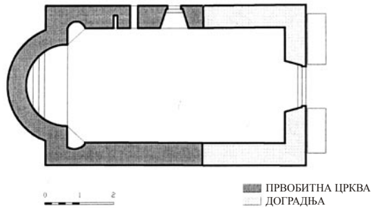
Основа цркве св. Неђеље у Кумбору
